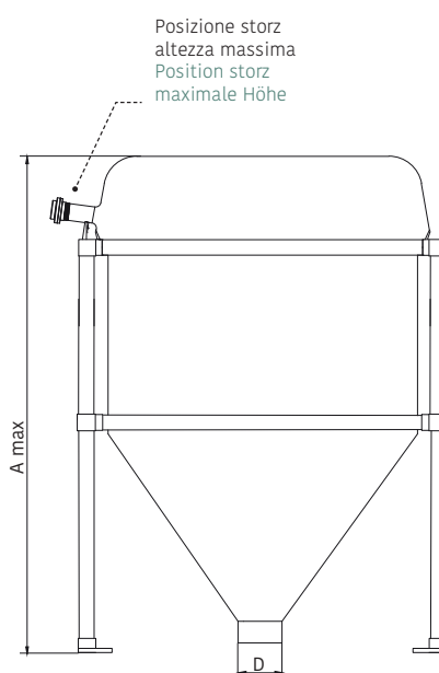
VISTA FRONTALE/FRONTANSICHT
